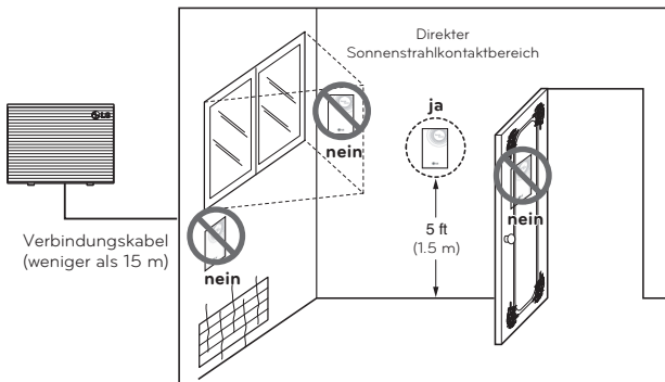
Fernlufttemperatursensor
