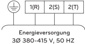
Klemmleiste 2 (in 3Ø Zusatzheizung)
